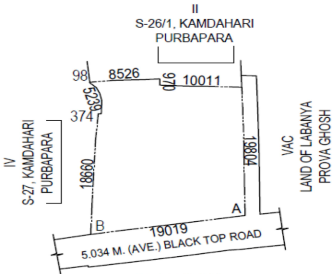
SITE PLAN (SCALE - 1 : 600)
